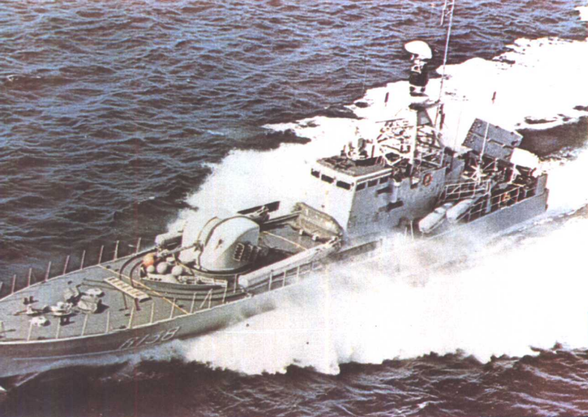
瑞典诺尔彻平级导弹艇
