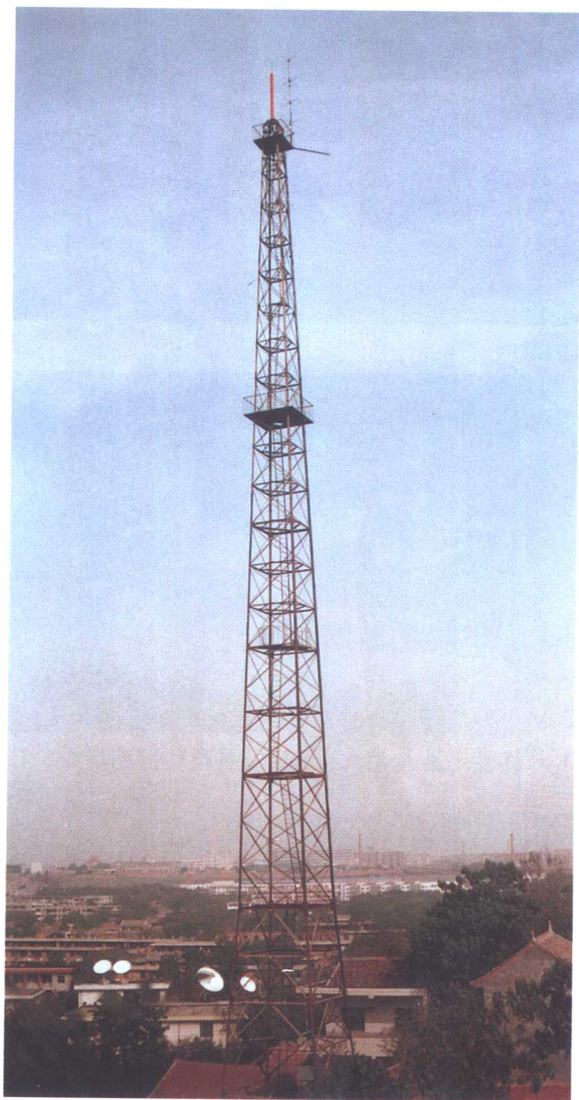
长安县广播电视调频发射塔(韦曲)
