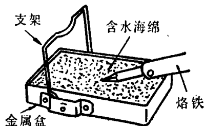
图1—4 烙铁除垢器
