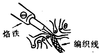
图1—3 用编织线沾焊锡
