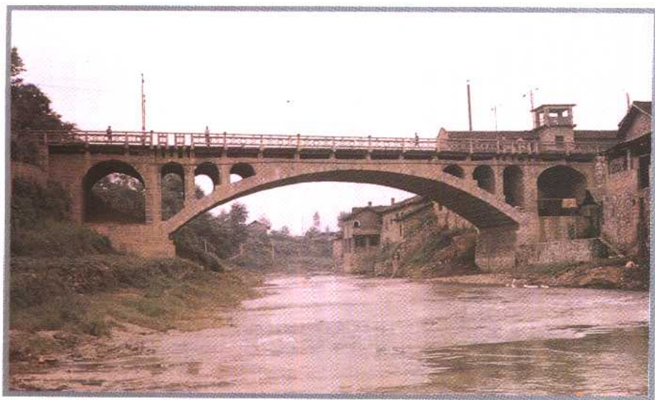
玉溪大桥
