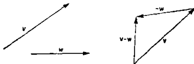
图 6 向量减法
