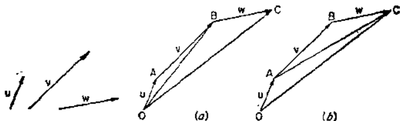
图 4 结合律: (\mathbf{u} + \mathbf{v}) + \mathbf{w} = \mathbf{u} + (\mathbf{v} + \mathbf{w})
