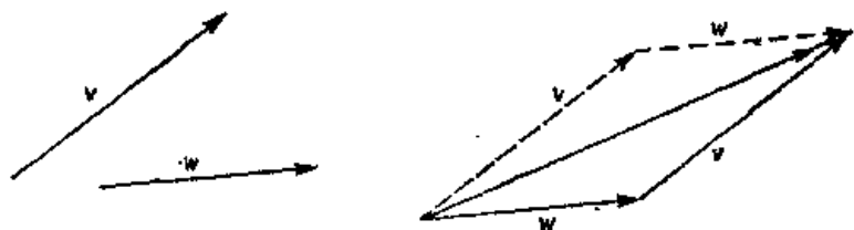
图 3 交换率: \mathbf{v} + \mathbf{w} = \mathbf{w} + \mathbf{v}
