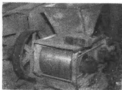
土法榨油使用的花生剥壳机。
