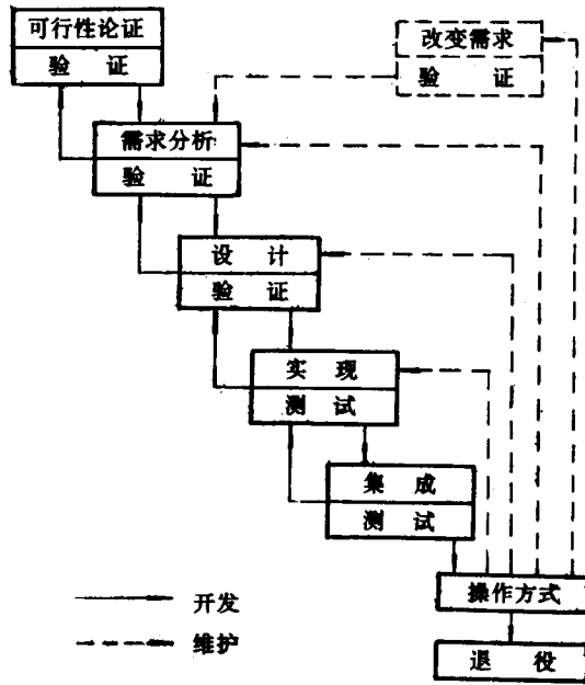
图 1.2 瀑布模型
