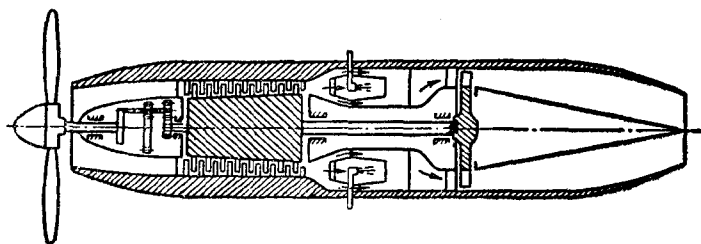
圖 2. 氣輪螺旋式發動機簡圖。
