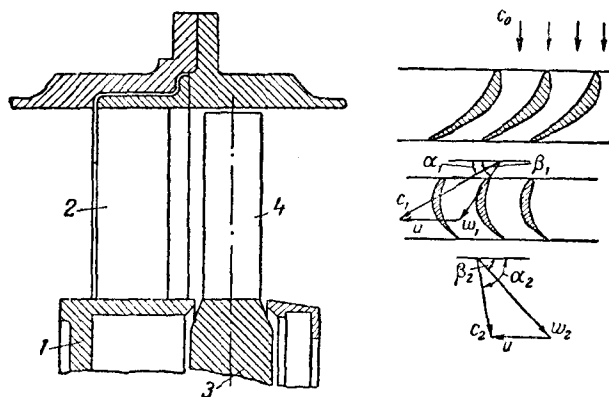
圖 3. 軸流式氣輪機的流程部分。
