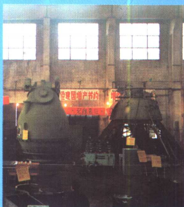
1260M 3 高炉原料钟顶设备
