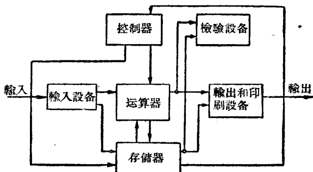
图3 电子数字计算机的方框图。
