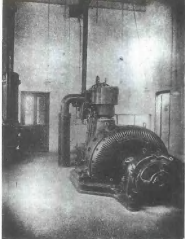
常州第一台 180 千瓦 发电机组 (1914 年)
