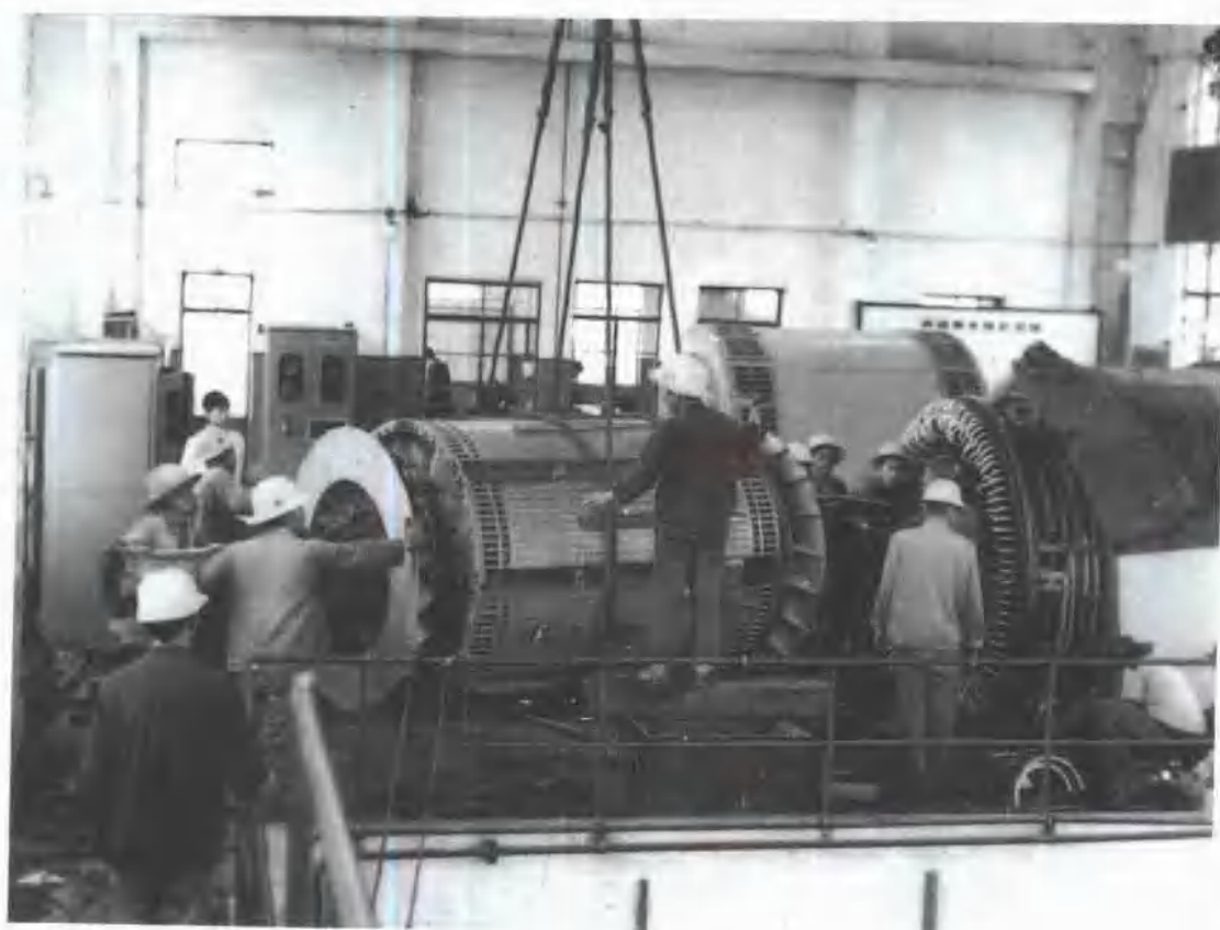
常州供电局2号调相机改装工程
