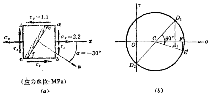
图 10-7 例题 10-2 图
