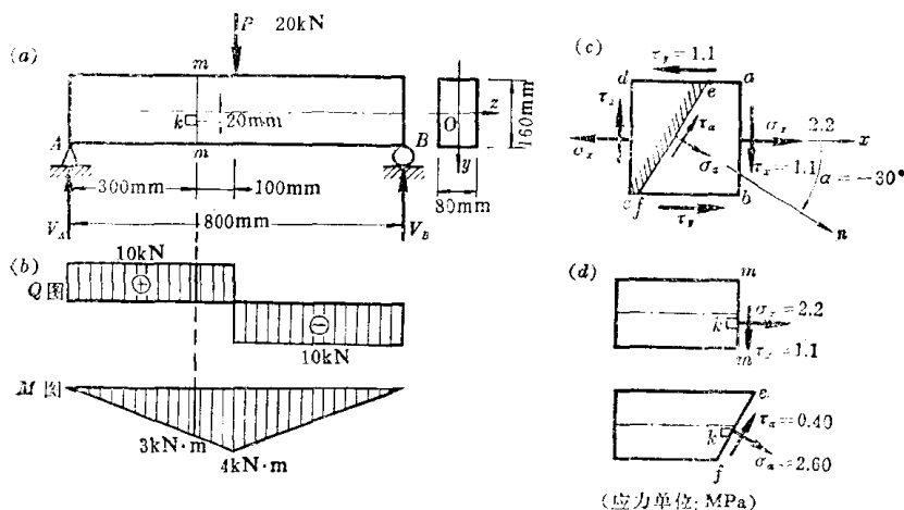
图 10-5 例题 10-1 图
