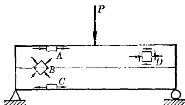
图 10-2 横力弯曲杆中点的应力状态
