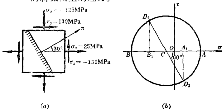
图 10-8 例题 10-3 图
