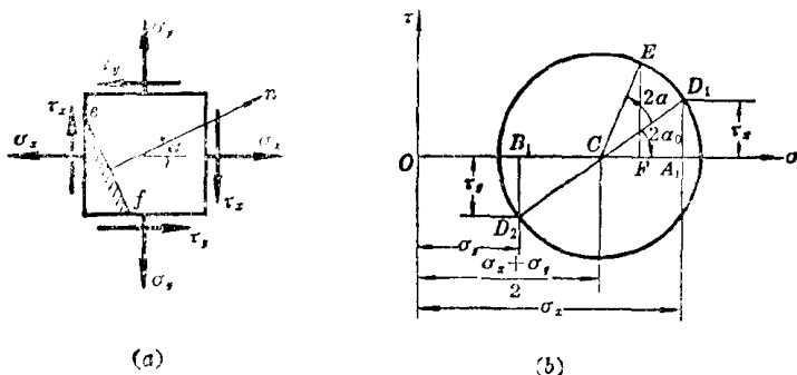
图 10-6 应力圆
