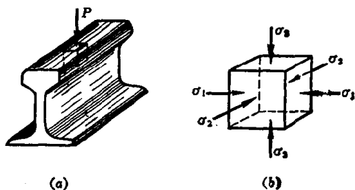
图 10-3 三向应力状态的例子
