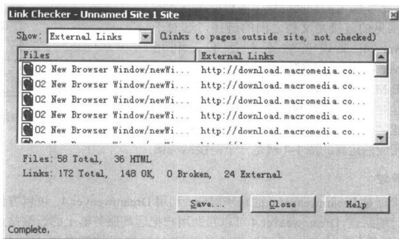
图1-5 检查链接
