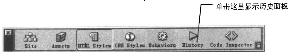
图1-2 控制栏
