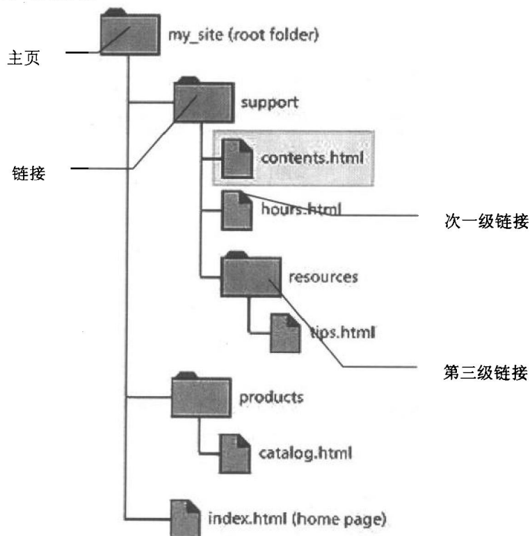
图1-4 链接结构图
