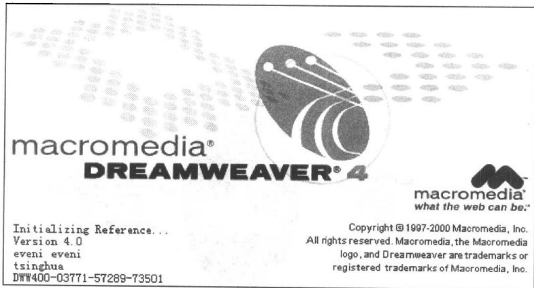
图1-1 Dreamweaver 4主界面
