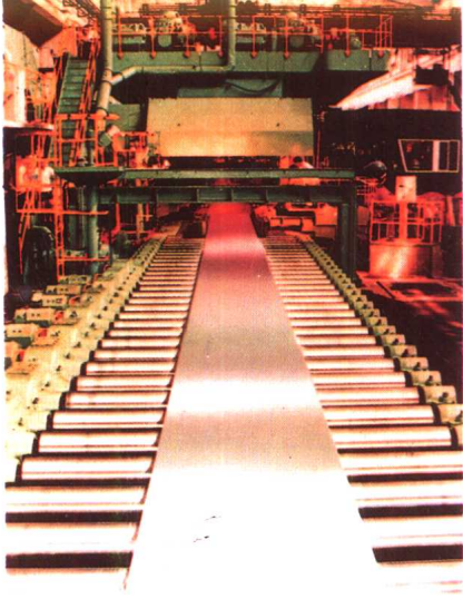
西南铝加工厂国产 2800 毫米铝板轧制生产线
