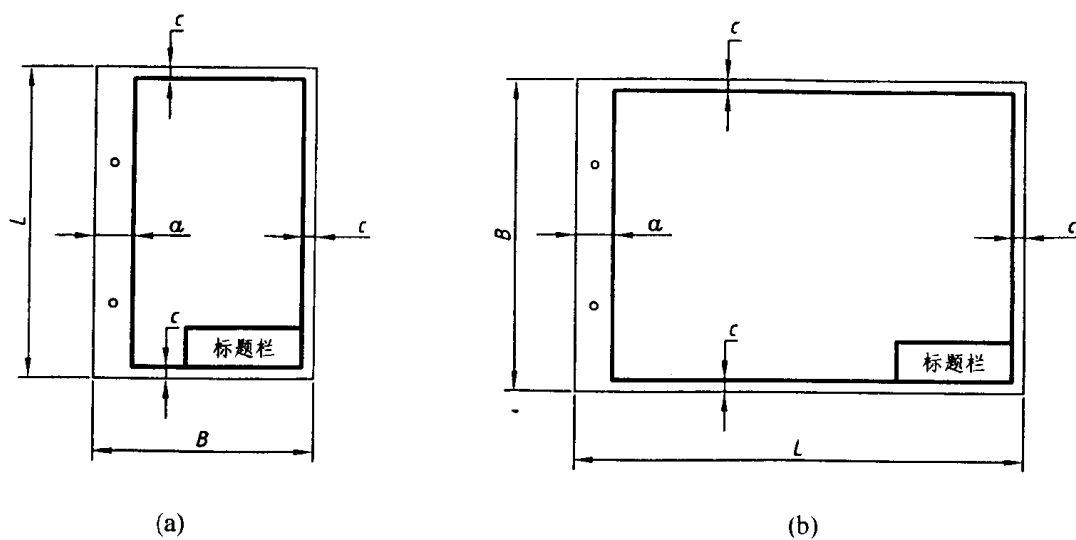
图 1-3 留有装订边的图框格式
