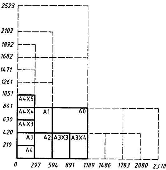
图 1-1 图纸基本幅面及加长幅面尺寸
