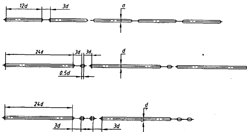
图 1-9 图线的构成
