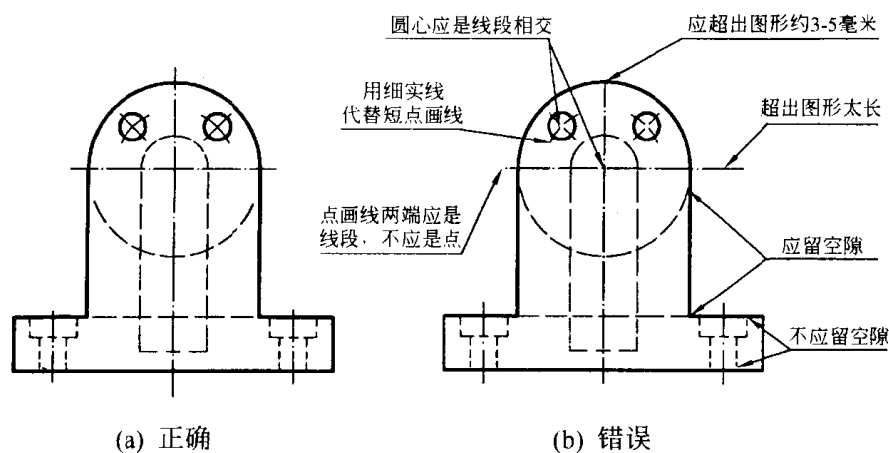
图 1-11 图线画法示例
