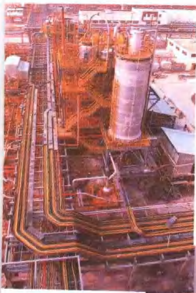
辽宁盘锦天然气化工 4万吨/年聚丙烯装置
