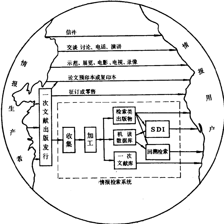
图1-1 情报流程图
