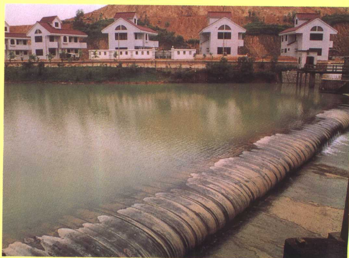
洪秀全水库橡皮坝
