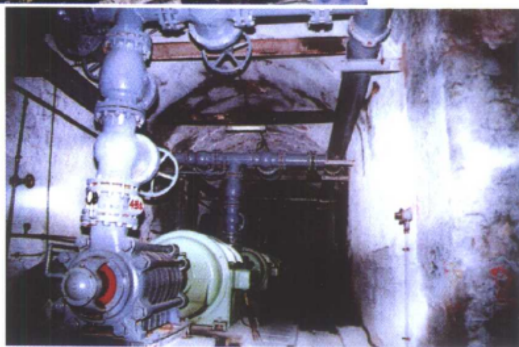
煤矿井下水泵房
