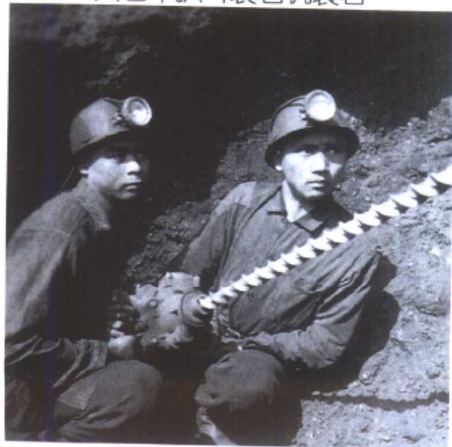
回采工作面打炮眼
