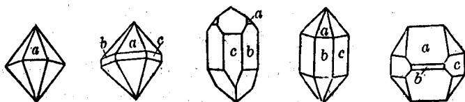
图 1-3 石英晶体的若干外形
