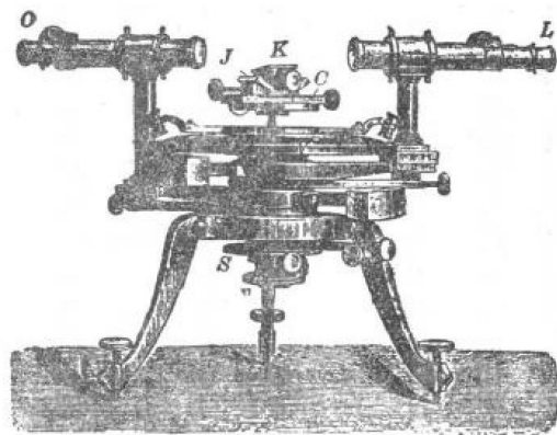
圖一〇 反射測角器之一例
