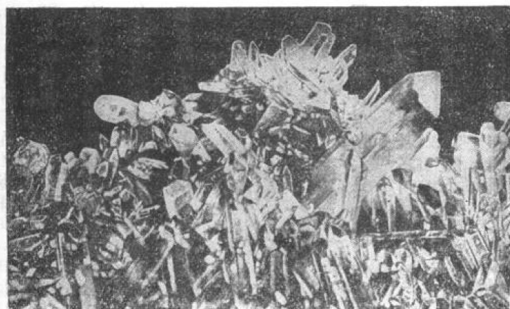
圖二 水晶之結晶羣
