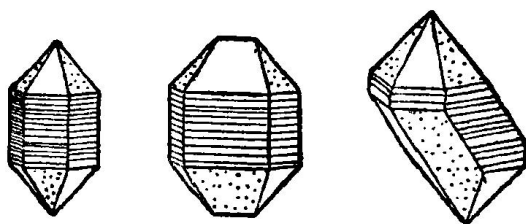
圖六 水晶之種種
