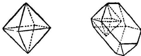
圖七 螢石之結晶
