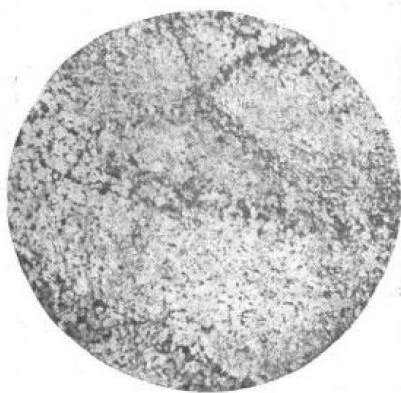
圖三 黃鐵礦之集合
