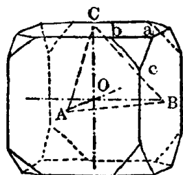
圖一 軸率之選定
