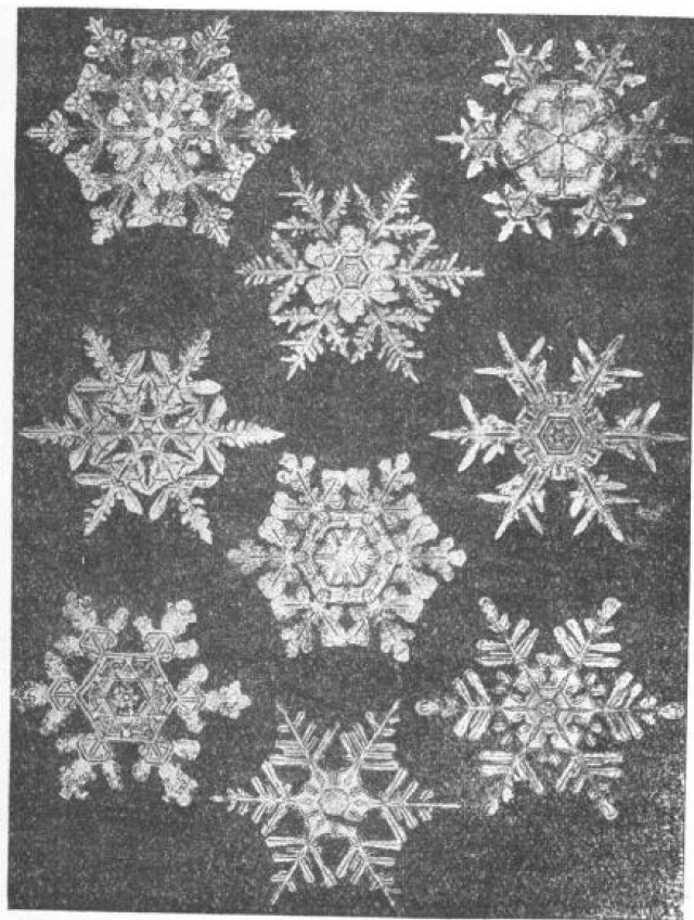
圖一 雪之結晶
