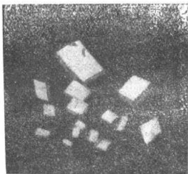
圖四 方解石之劈開
