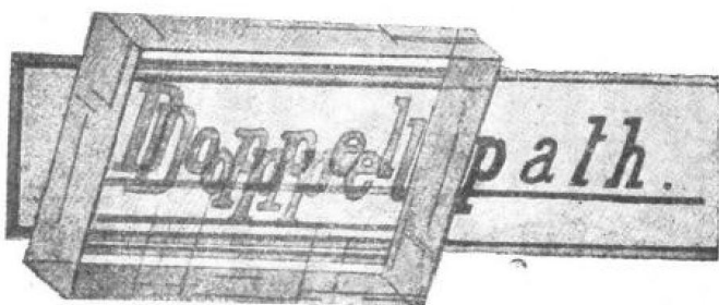
圖五 方解石之重屈折
