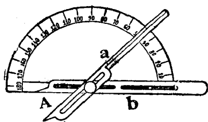
圖八 接觸測角器
