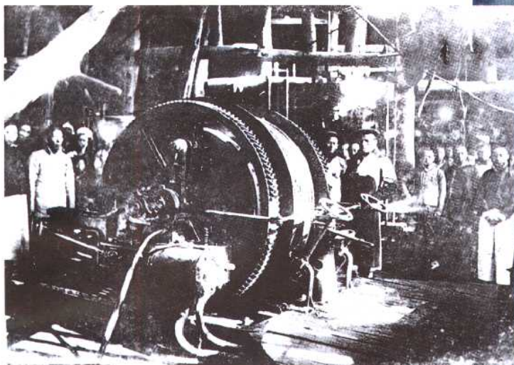
蒸汽卷扬机采卤
