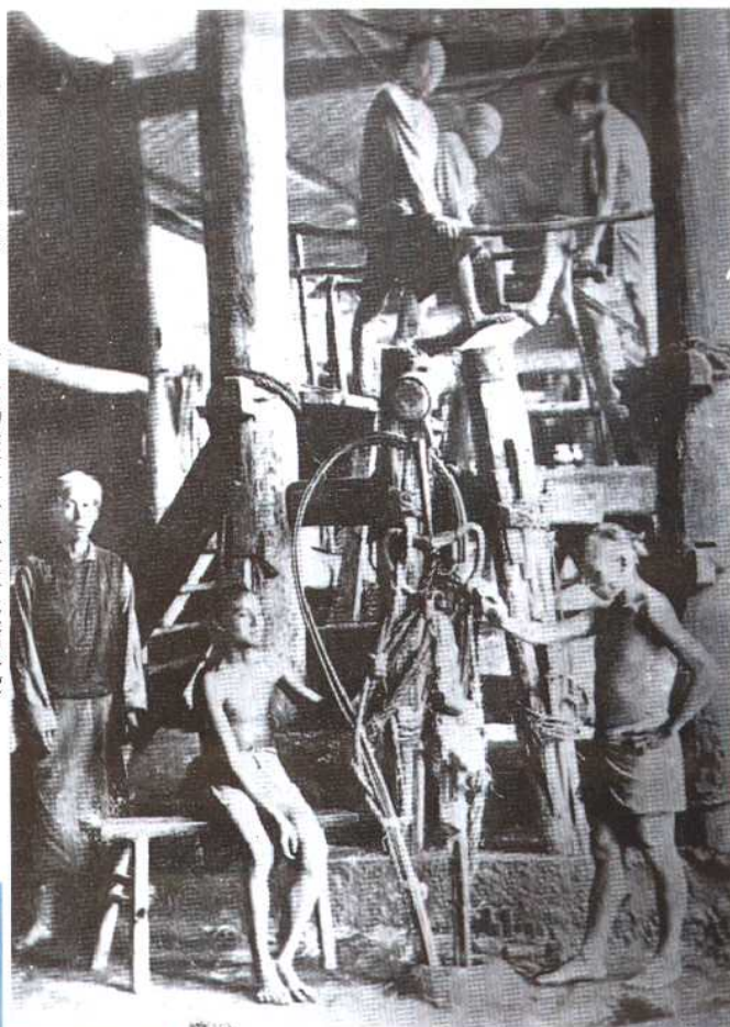
世界上第一口超千米深井——柴海井（凿于1835年）
