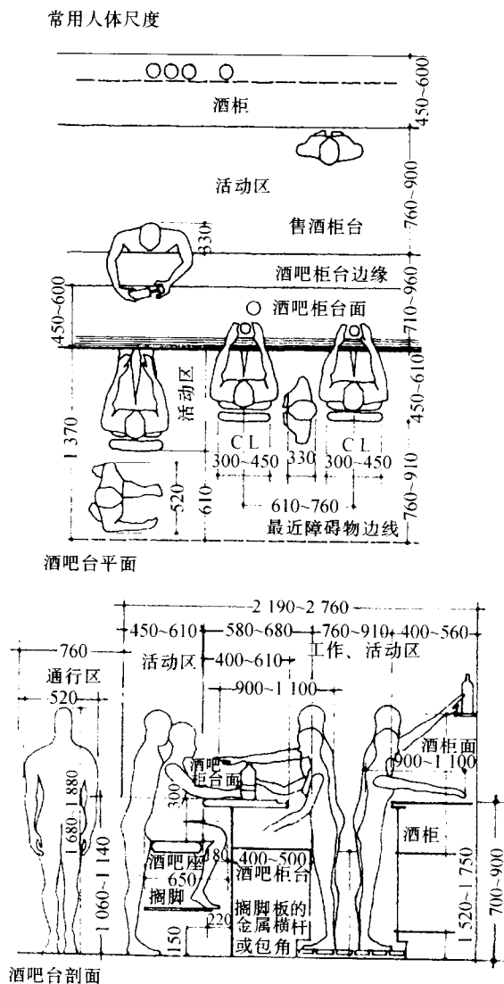
图 8-1 人体尺度与酒吧台平面、剖面关系
