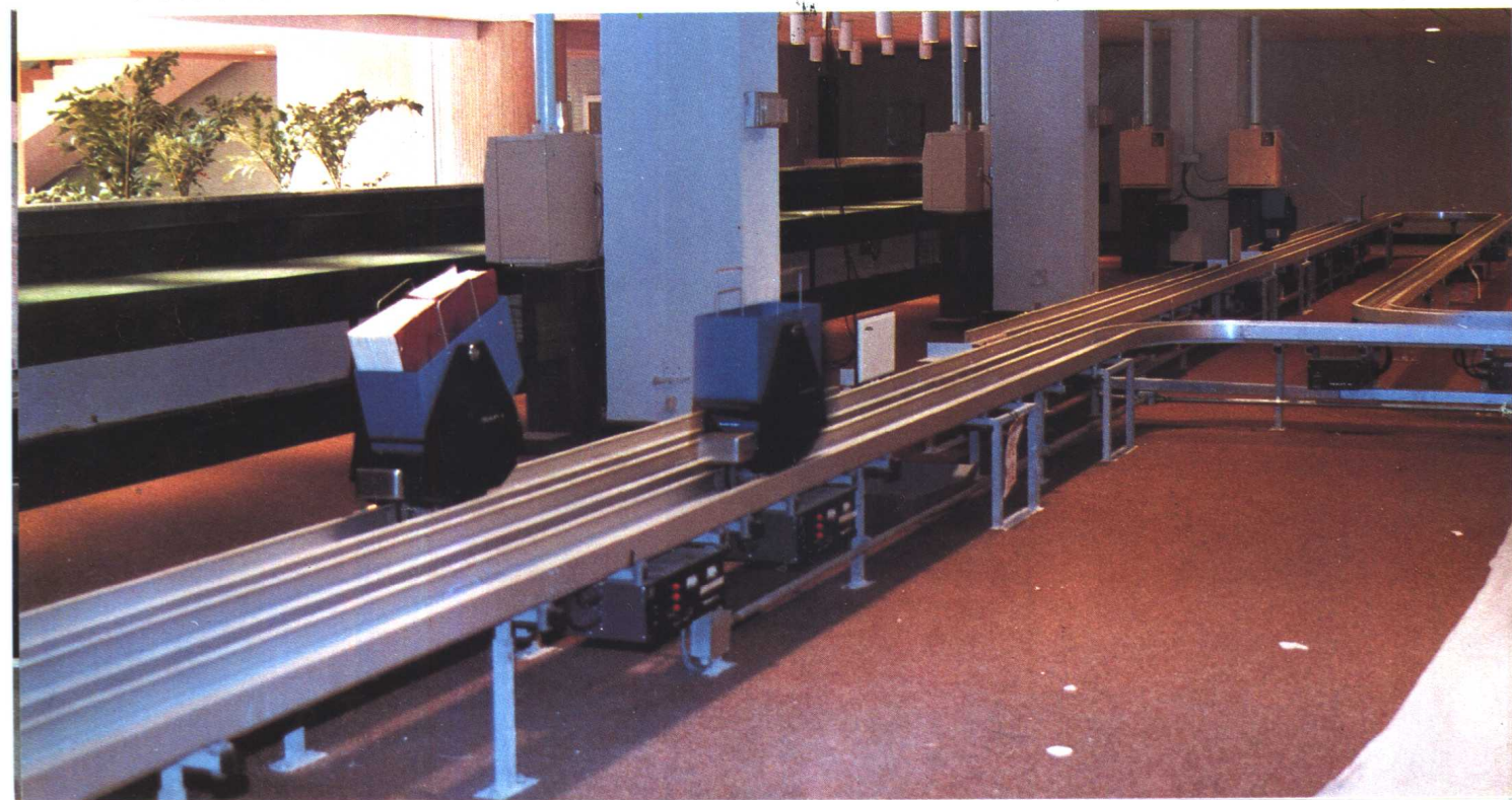
基本书库书刊自走台车传送设备
