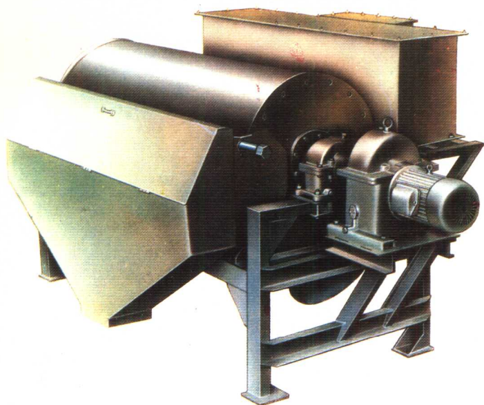
CT——1024 永磁筒式磁选机是沈阳矿山机器厂的产品，适用于湿式选别细颗粒强磁性矿物，1984年获国家银质奖。
