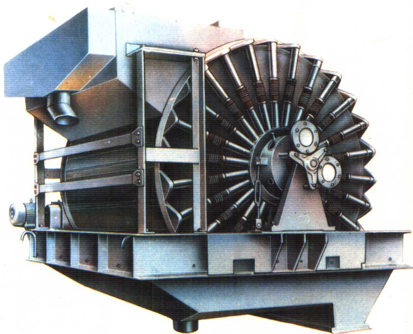
沈阳矿山机器厂生产的GYW型真空永磁过滤机，1982年获机械工业部优质产品。
