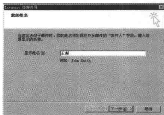
图 1-3 输入姓名
