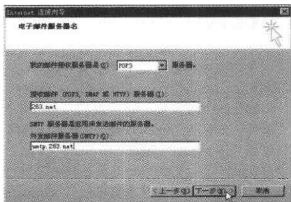
图 1-5 输入收发邮件服务器地址
