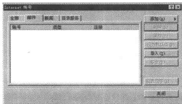
图 1-2 添加新账号
