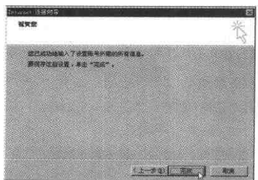
图 1-7 完成设置
