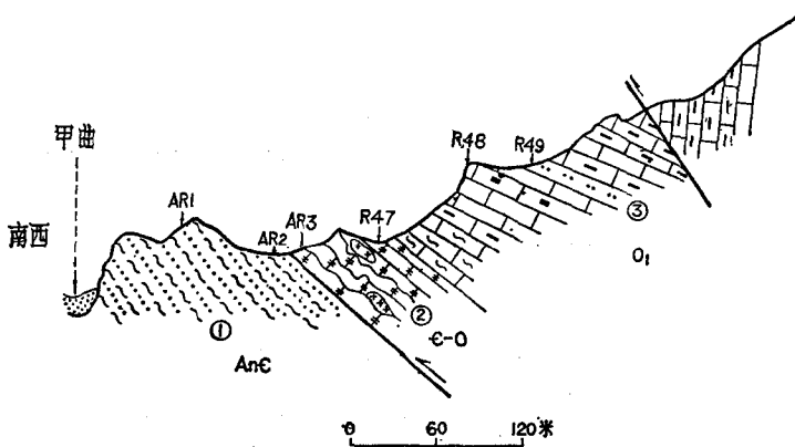
图 2-5. 甲村东北山坡地层剖面示意图
