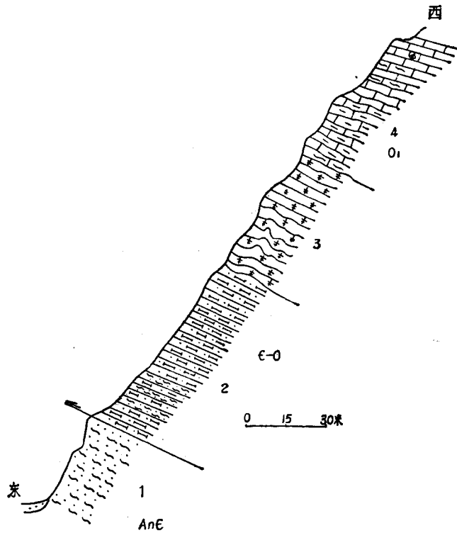
图 2-2. 聂拉木县肉切村西北沟肉切村群剖面示意图 1. 珠穆朗玛群; 2. 肉切村群下组; 3. 肉切村群上组; 4. 甲村群上组。
