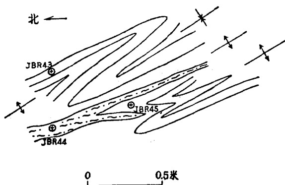
图 2-4. 定日—聂拉木公路十二道班房西山肉切村群下 组石英片岩构成的紧闭褶曲素描 (JBR43.方解石石英片岩; JBR44.长英质糜棱岩; JBR45.透辉石石英片岩。)
