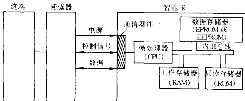
图 1.2 智能卡的芯片结构
