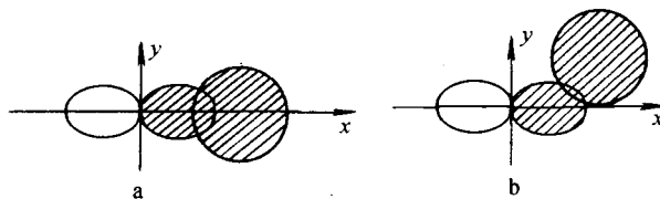
图 1-2 s 轨道和 p 轨道的重叠
