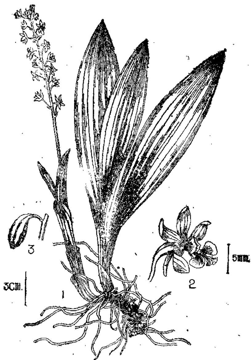
图2. 九子莲 Calanthe discolor Lindl. 1. 植物全株 2. 花 3. 果
