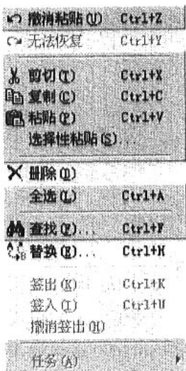
图 1-12 “编辑”菜单
