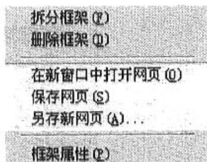
图 1-18 “框架”菜单
