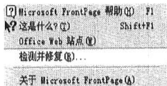
图 1-20 “帮助”菜单
