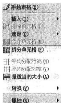
图 1-17 “表格”菜单
