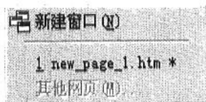
图 1-19 “窗口”菜单
