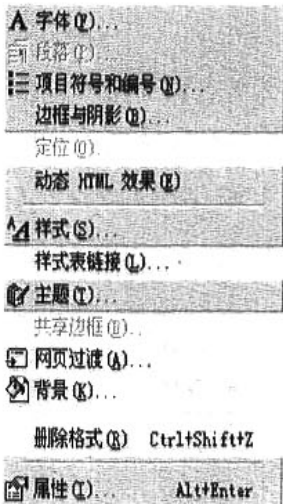
图 1-15 “格式”菜单
