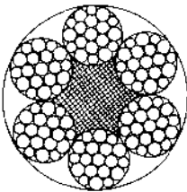
6×19W+FC 直径 6~40mm
