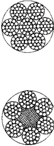
第 2 组 6×19(b)类
