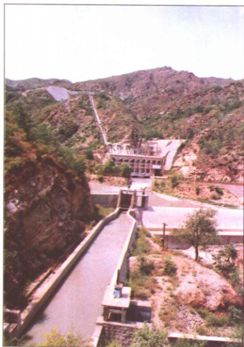
紫荆关梯级水电站, 图为三级电站
