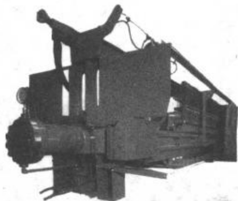
厢式程控自动压滤机
