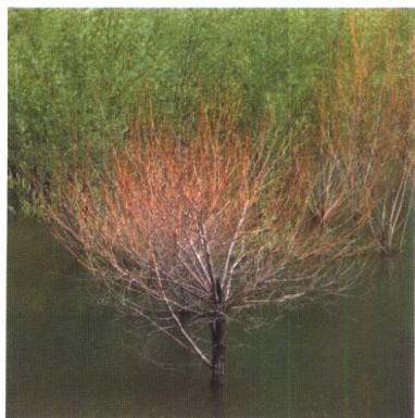
红柳树
