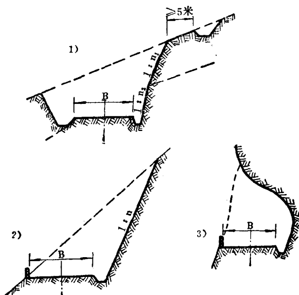
图1-2 挖方路基典型断面图
