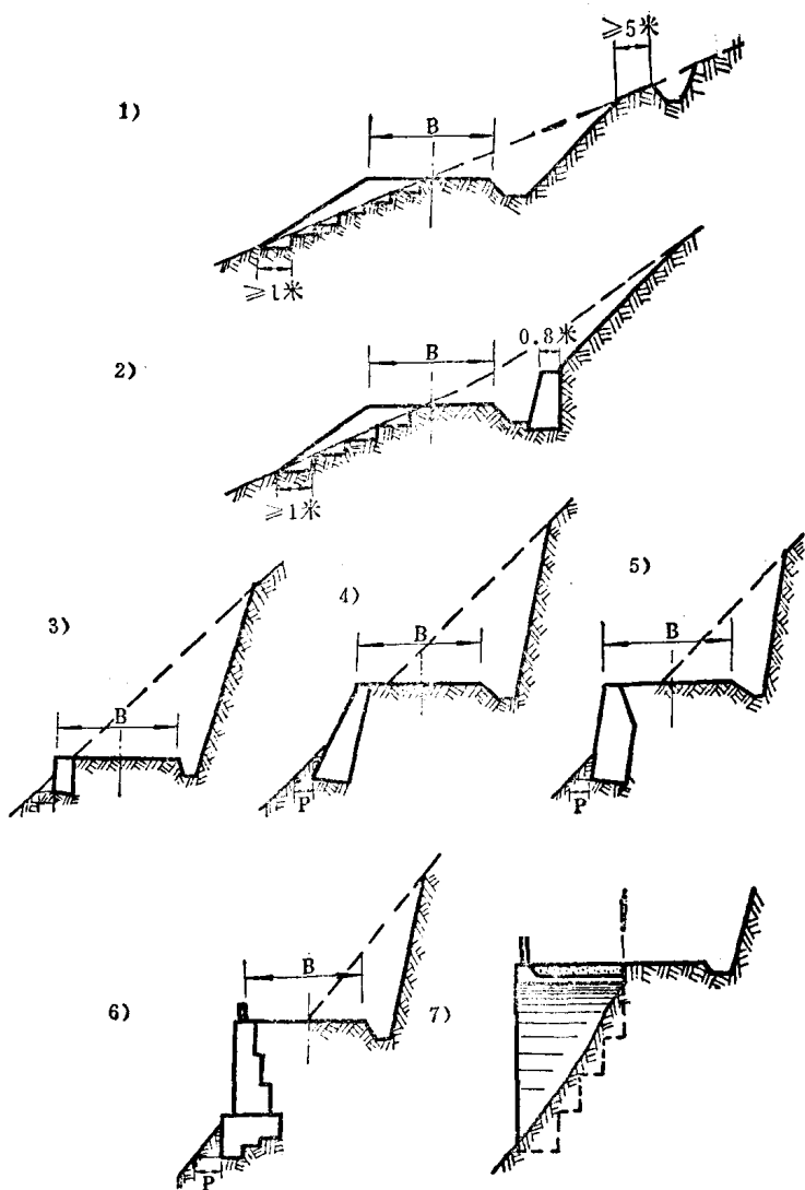
图1-3 半挖半填路基典型断面图
