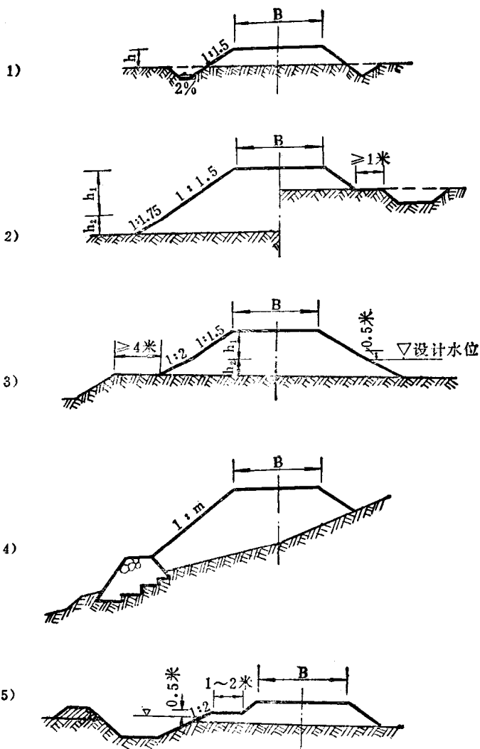
图1-1 填方路基典型断面图
