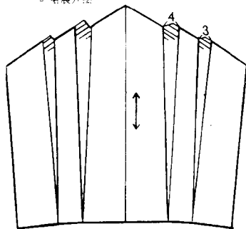
前裙展开图
