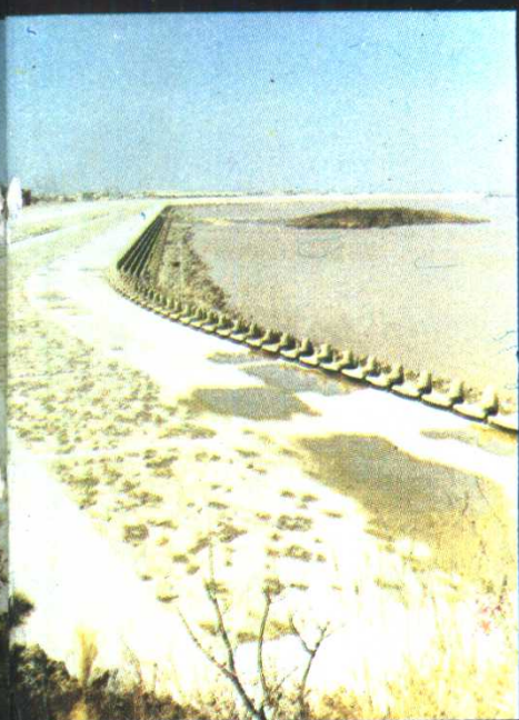
秦山核电厂配套工程——扩岸拦海大堤
