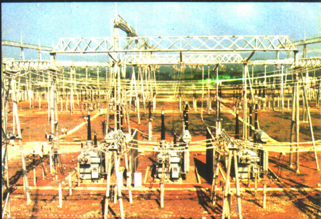
我省第一座50万伏的杭州瓶窑变电所外景
