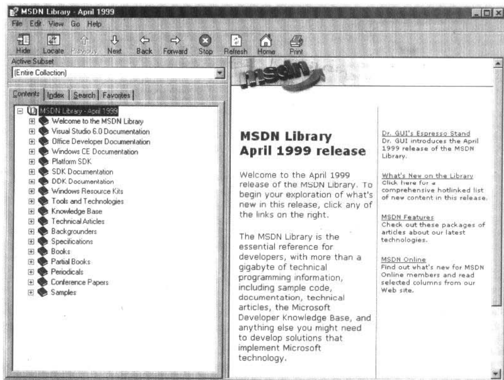
图3-2 MSDN界面
