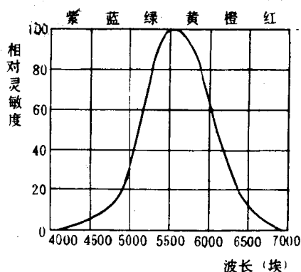
图 1-1 视觉相对灵敏度与波长的关系
