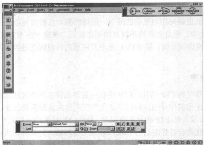
图 1-3 Dreamweaver 界面
