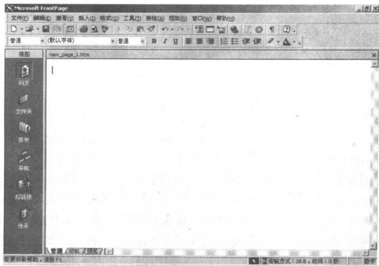
图 1-4 FrontPage 界面
