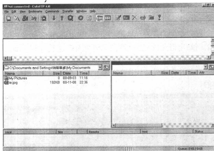
图 1-5 CuteFTP 界面
