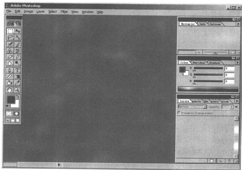
图 1-7 Photoshop 界面
