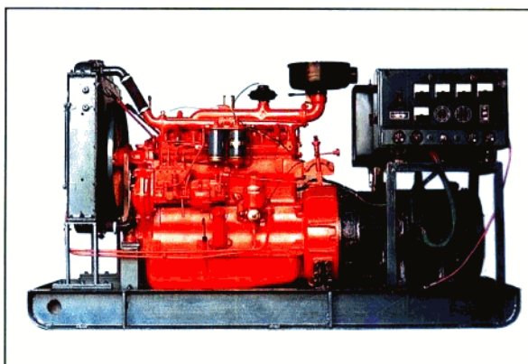
GF 系列 30KW 交流工频柴油发电机组
