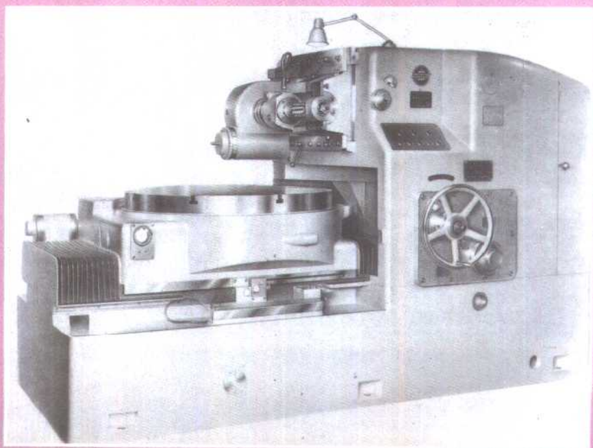
▲1967年，重庆机床厂生产的我国第一台自行设计YG3780型高精度蜗轮滚齿机，1978年获全国科学大会科技成果奖
