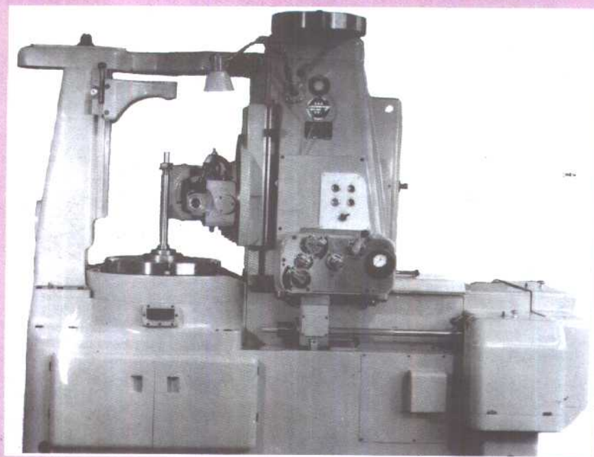
▲1953年，重庆机床厂试制成功并投产的 我国第一台Y37型滚齿机
