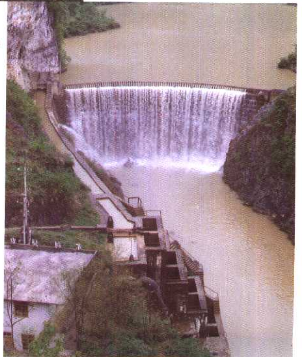
全国扬程最高的新民水轮泵站 ▶
