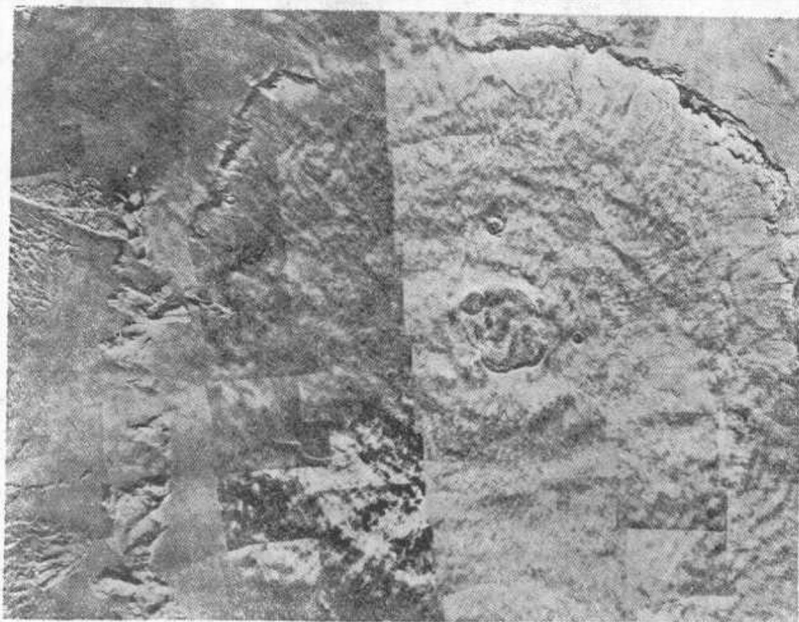
火星上的地理特征使地球上的类似特征相形见绌。马利诺斯德大峡谷看上去像一条壕沟。奥林匹斯火山(下图)是火星上
