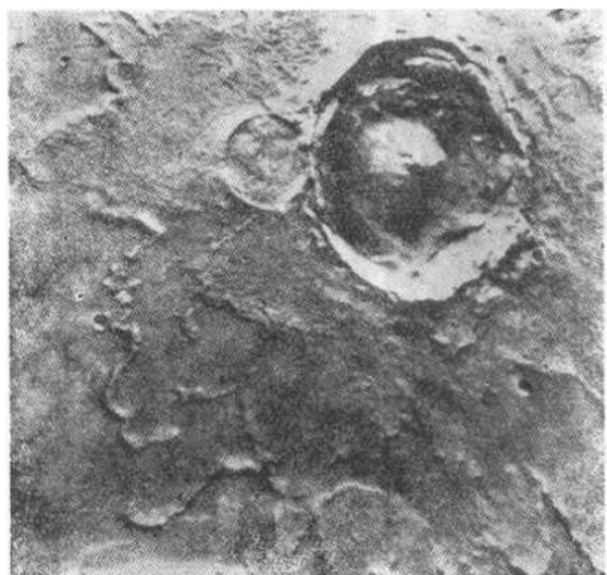
尤蒂坑(Yuty crater)大概是陨星与火星碰撞造成的。破碎的岩石,由于冲击力的作用,一层层被抛向坑口周围
