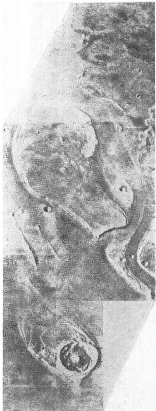
火星克赖斯平原上的珠状“海岛”，位于曲折的、纵横交错的河道当中，它是水在那里一度奔流过的有力迹证
