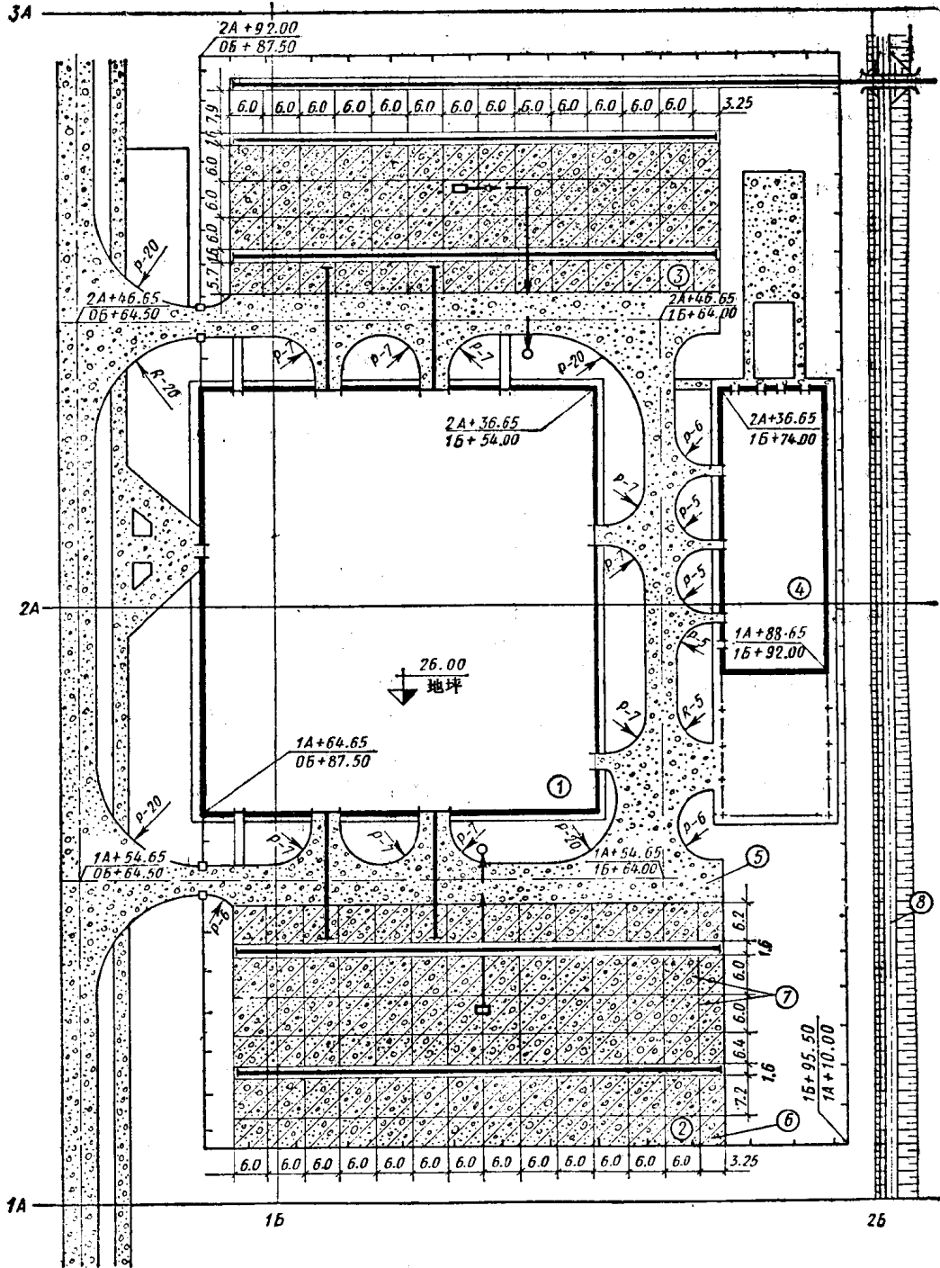
图10 厂区内公路平面图
