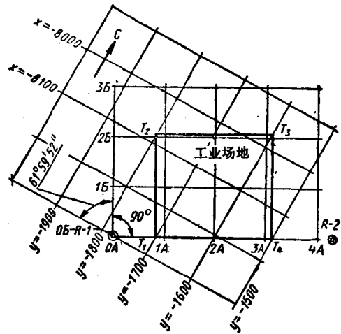
图6 建筑方格网关系图
