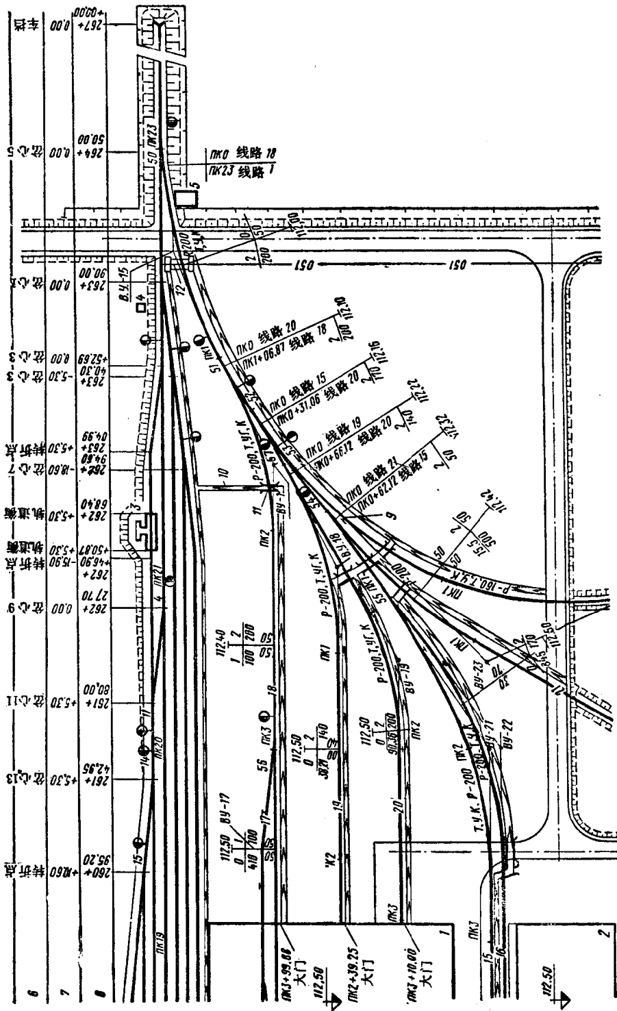
图9 厂区内铁路平面图 1~5—建筑物和构筑物 6—线路点名 7—与基线距离 8—百米标或座标 9—曲线终点或起点 10—排水沟 11—排水涵管 12—雨水井 P—曲线半径 T—曲线切线长 Y—曲线转向角 R—曲线长度
