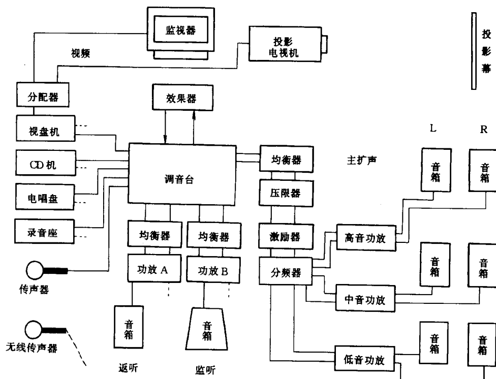
图 0-2 厅堂扩声系统的基本组成框图
