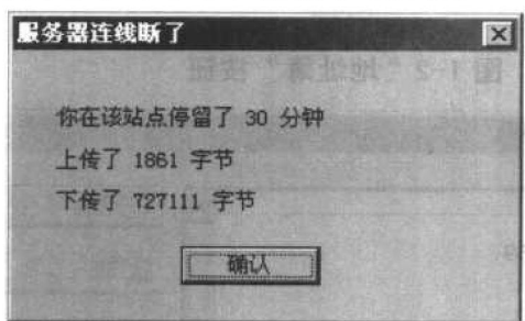
图 1-4 断开信息
