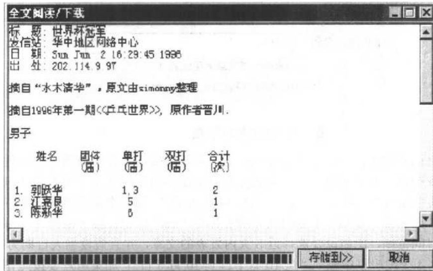
图 1-5 拷贝全文
