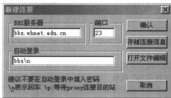
图 1-1 新建连接
