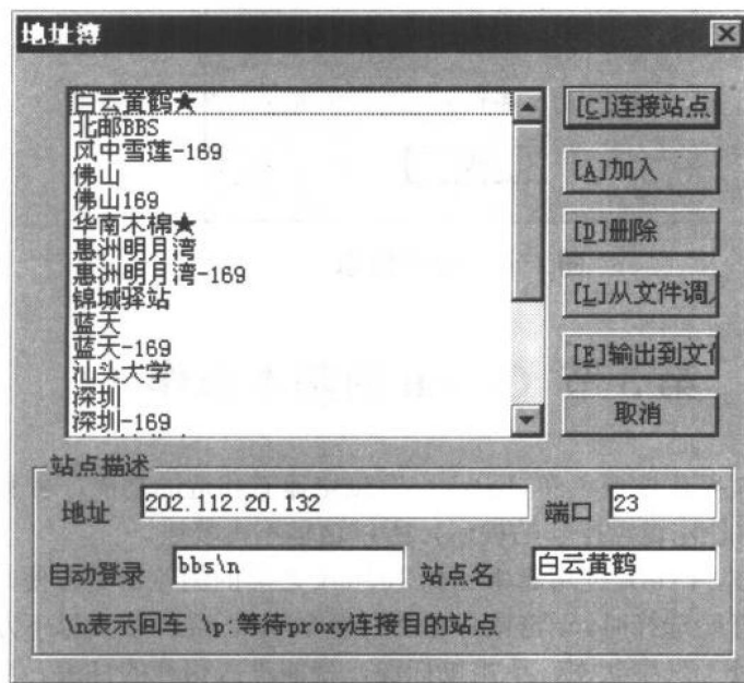
图 1-3 地址簿
