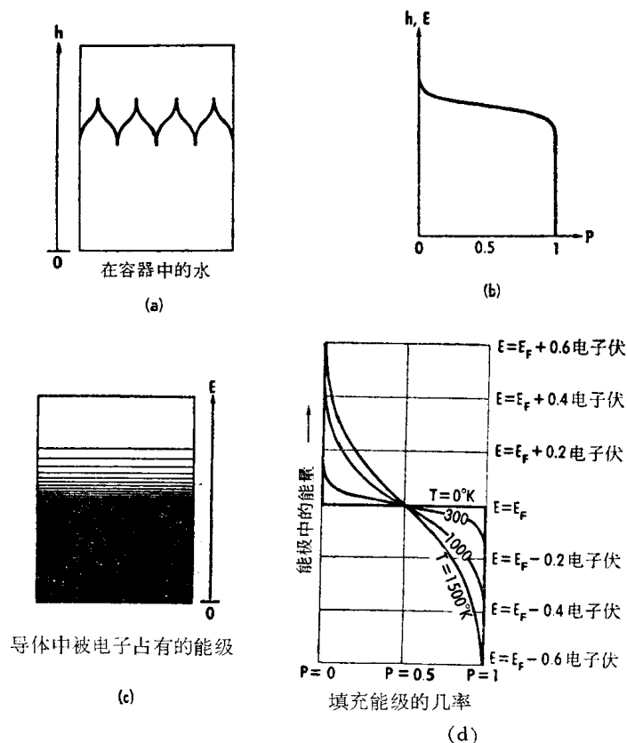
图 1-3 (a) 容器中的水被搅动时的情况; (b) 在各种不同高度 (能级) 时水 (电子) 的存在几率; (c) 导体中被电 子占据的能级; (d) 四种不同温度时的费米分布函数。 (引自参考书目 2)
