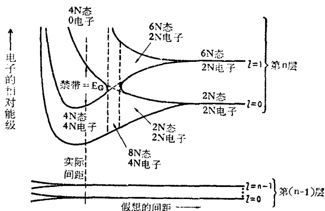
图 1-2 金刚石结构的理论能级与原子间距的关系。
