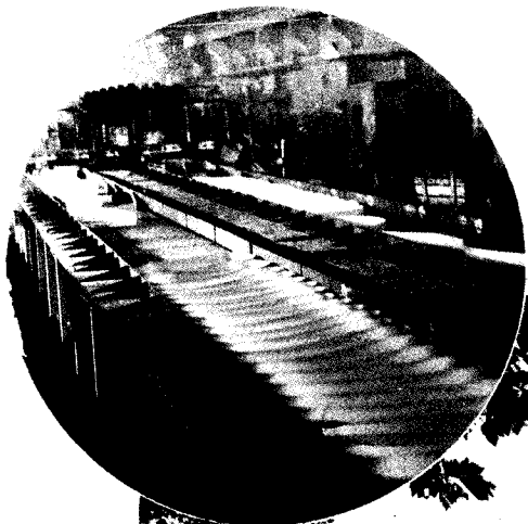
◀ 图为该厂自行设计、制造的我国第一套具有先进水平的450毫米四分之三热连轧窄卷带机组。
